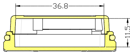
剖面 H-H
